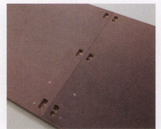
RBT-11の天板連結構造
